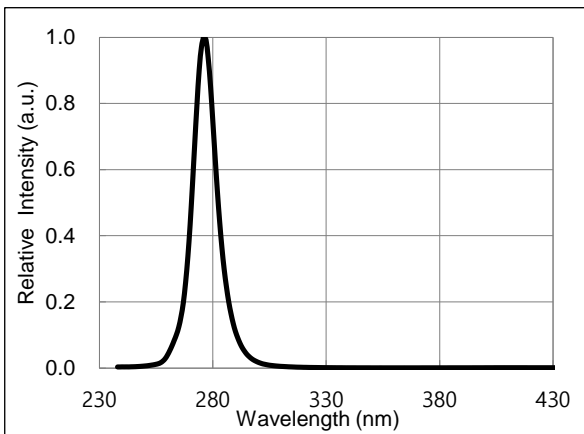
Spectrum, T_a=25^\circ\text{C} , I_F=150\text{mA}
