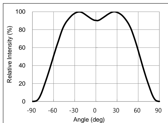
Beam Angle, T_a=25^\circ\text{C} , I_F=100\text{mA}
