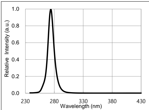
Spectrum, T_a=25^\circ\text{C} , I_F=100\text{mA}
