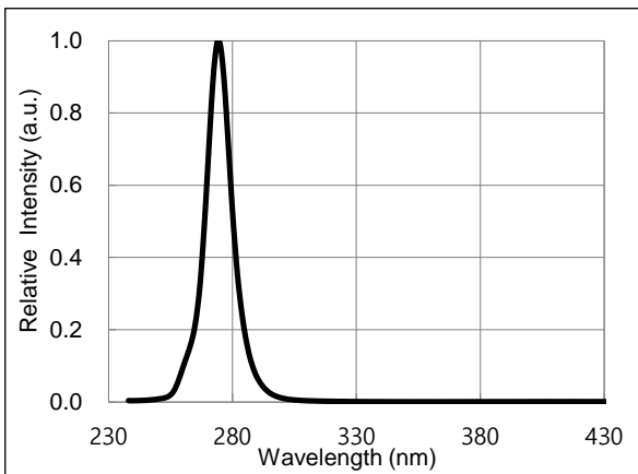
Spectrum, T_a=25^\circ\text{C} , I_F=20\text{mA}
